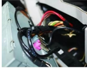
17. Ziehen Sie den Stecker des Original-Motorsteckers ab
