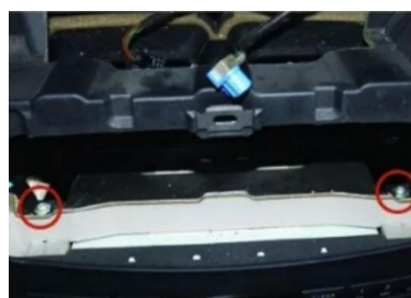
15. Lösen Sie die Schrauben des Originalmotors und drücken Sie ihn nach unten, um ihn herauszunehmen
